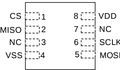
图 2-4 SQ7133 8-Lead DFN 封装型态引脚配置
