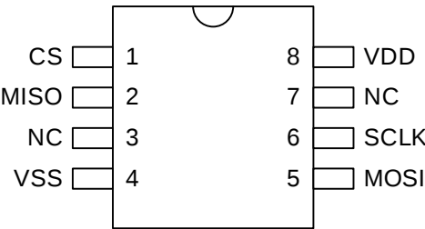
图 2-3 SQ7133 SOP8 封装型态引脚配置
